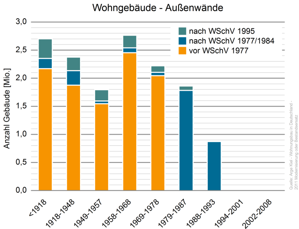
Abbildung 82: Energetisches Niveau der Außenwände der Gebäude in Deutschland
