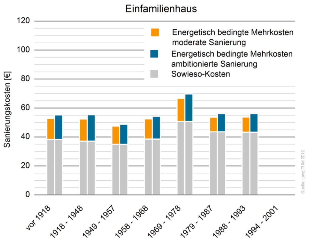
Abbildung 54: Energetisch bedingte Mehrkosten von Sanierungen
