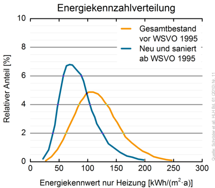
Abbildung 77: Energiekennzahlverteilung des Gebäudebestands und der sanierten Gebäude
