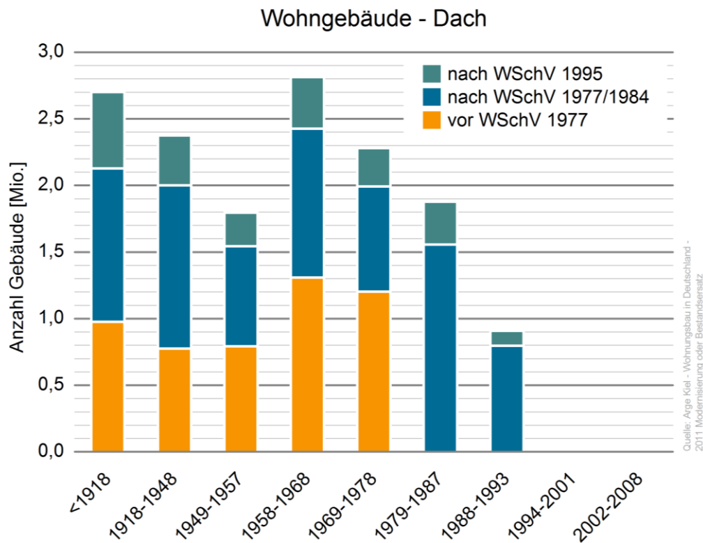
Abbildung 79: Energetisches Niveau der Dächer deutscher Gebäude
