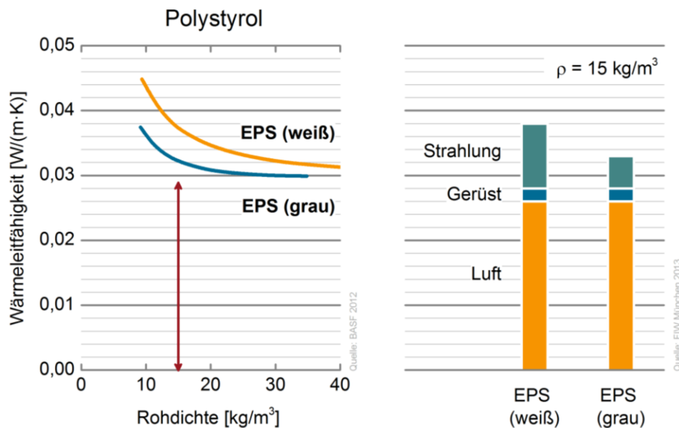
Abbildung 35: Innovationsprung bei Polystyrol - Einführung von grauem EPS
