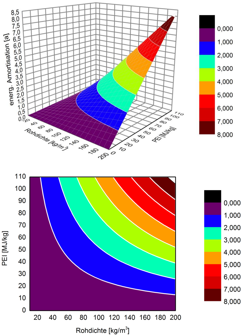
Abbildung 51: Energetische Amortisationszeit [a] als Funktion des Primärenergieinhalts [MJ/kg] und der Rohdichte [kg/m 3 ] bei konstanter Wärmeleitfähigkeit = 0,04 W/(m·K) und Dicke = 16 cm; als 3D-Plot (oben) und Darstellung der Isolinien (unten)
