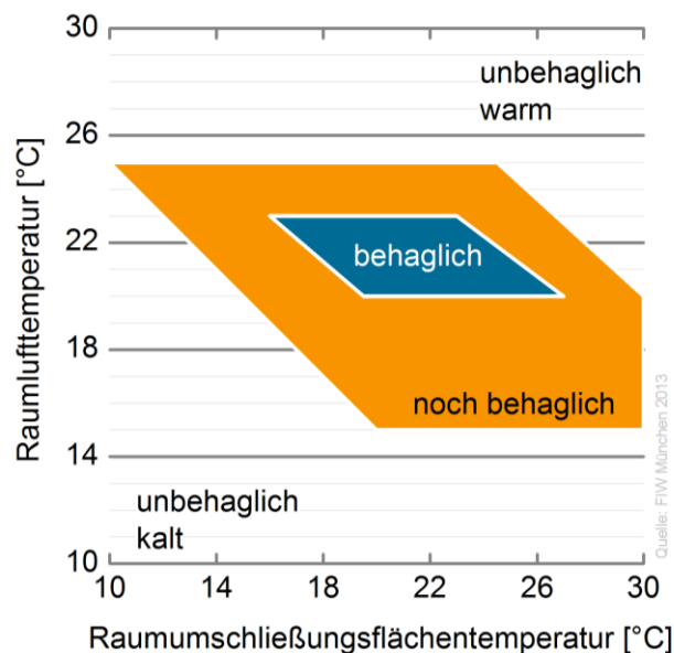
Abbildung 56: Behaglichkeitsfeld im Achsenkreuz von Raumlufttemperatur (Ordinate) und Temperatur der raumumschließenden Flächen (Abszisse) [Pistohl 1998]
