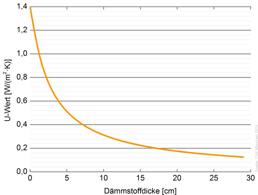
Abbildung 50: Einfluss der Dicke des Dämmstoffs ( \lambda = 0,04 W/(m·K)) auf den U-Wert eines Wandbauteils mit einem U-Wert des Rohbauteils von 1,4 W/(m²·K)
