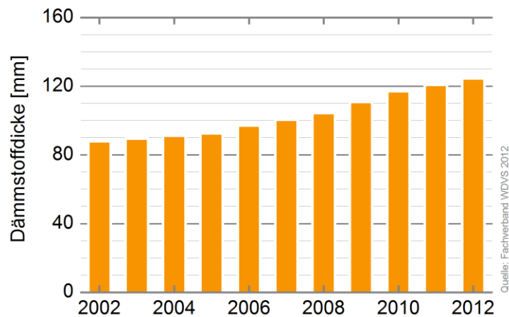
Abbildung 85: Zunahme der mittleren Dämmstoffdicke von WDV bei Sanierungen in Deutschland seit 2002
