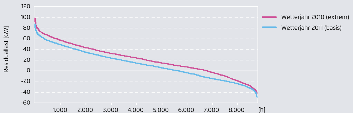
Jahresdauerlinie der Residuallast im Vergleich der Wetterjahre 2010 und 2011, Szenariojahr 2050
