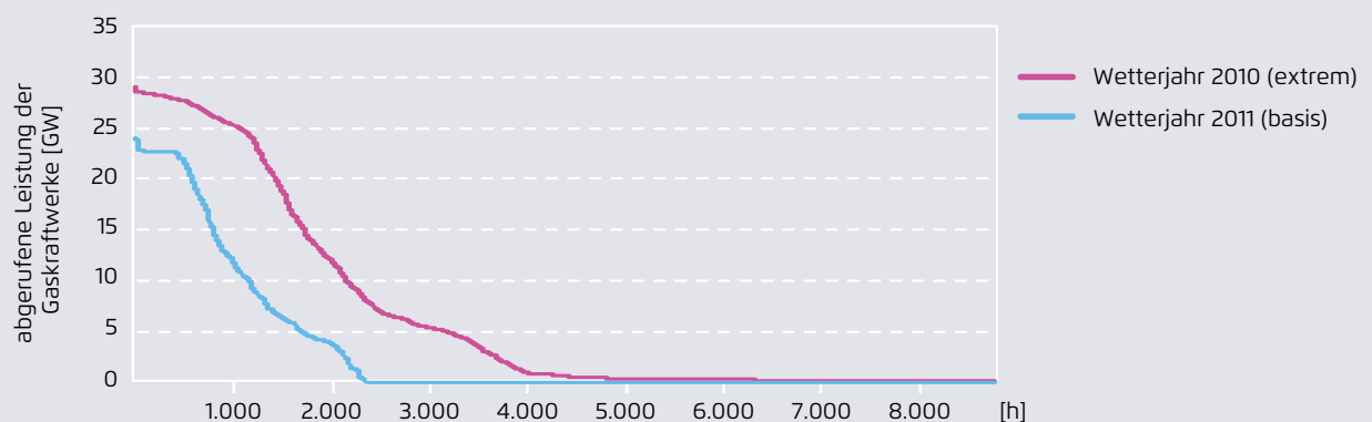
Jahresdauerlinien der Stromerzeugung aus Gaskraftwerken für die Wetterjahre 2010 und 2011, Szenariojahr 2050
