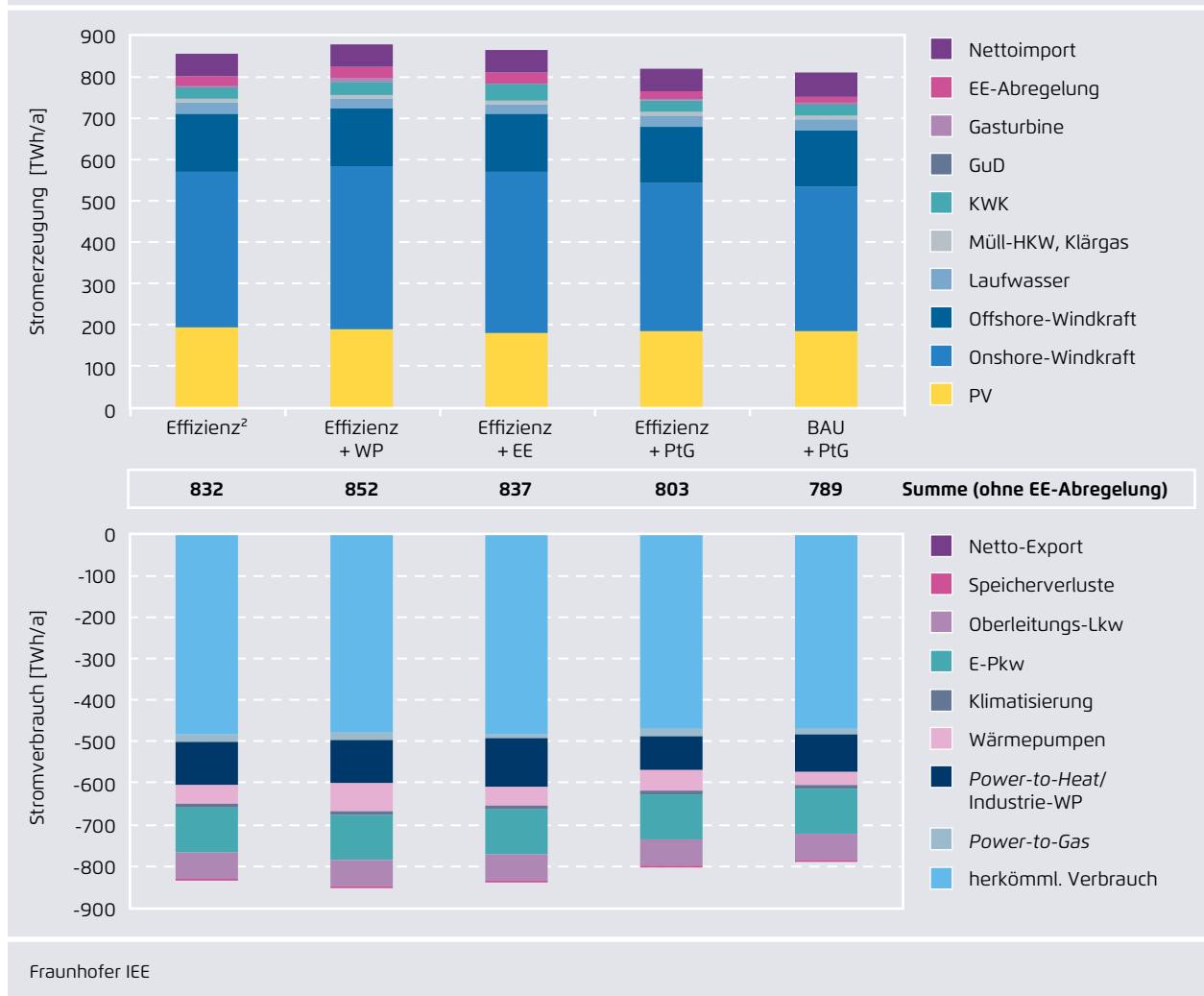
Vergleich der Stromerzeugung aufgelöst nach Anlagenart und des Stromverbrauchs aufgelöst nach Lastart
