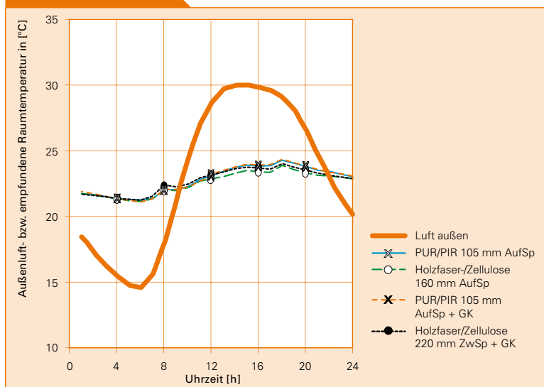
Außentemperatur und Raumlufttemperatur am heißesten Tag einer heißen Sommerwoche – mit Sonnenschutz
