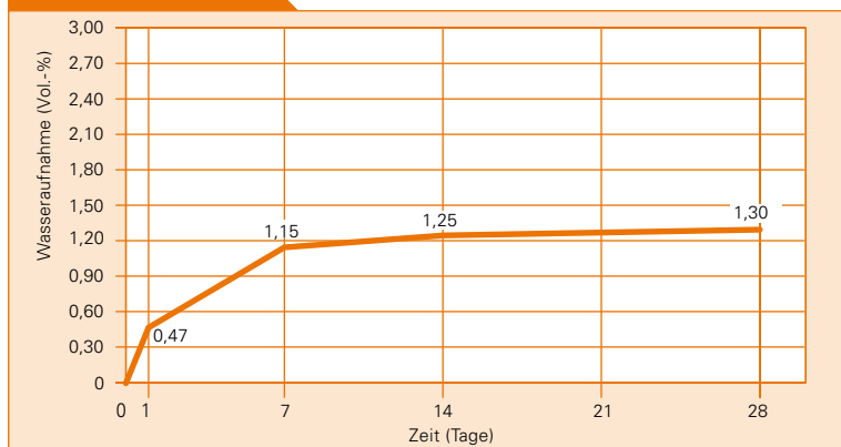
Wasseraufnahme von Polyurethan-Hartschaum nach 28-tägiger Unterwasserlagerung [3]
