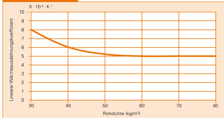
Thermische Ausdehnung von unkaschiertem PUR/PIR-Hartschaum im Temperaturbereich von -60^\circ\text{C} bis +20^\circ\text{C} in Abhängigkeit von der Rohdichte.
