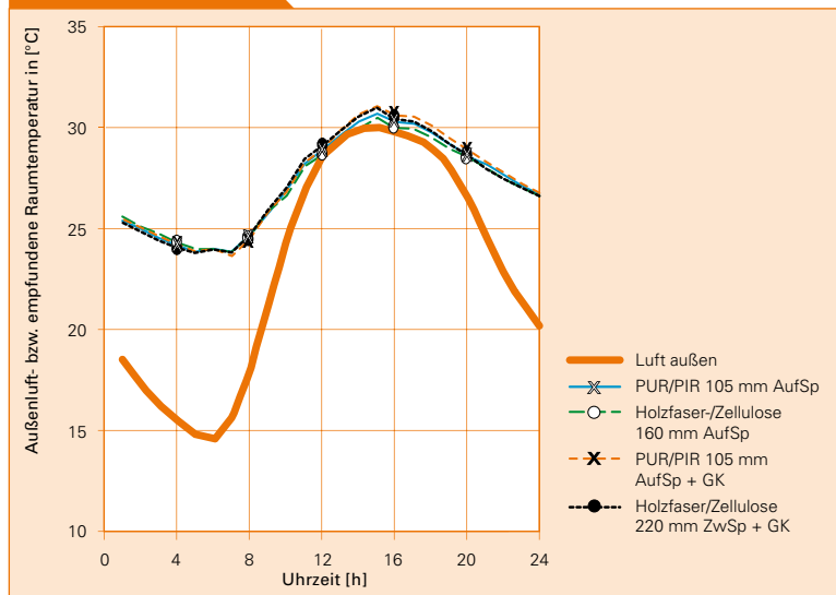
Außentemperatur und Raumlufttemperatur am heißesten Tag einer heißen Sommerwoche – ohne Sonnenschutz
